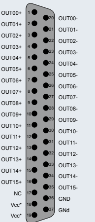
D-Sub-Buchse P1
