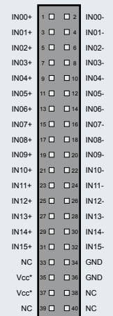
Pfostenstecker P2
