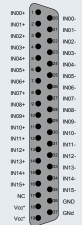
P2 als D-Sub-Buchse (optional)
