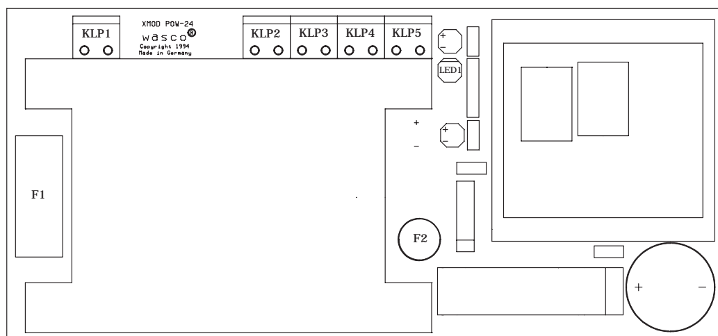
Abb.1-1 Komponentenlayout
