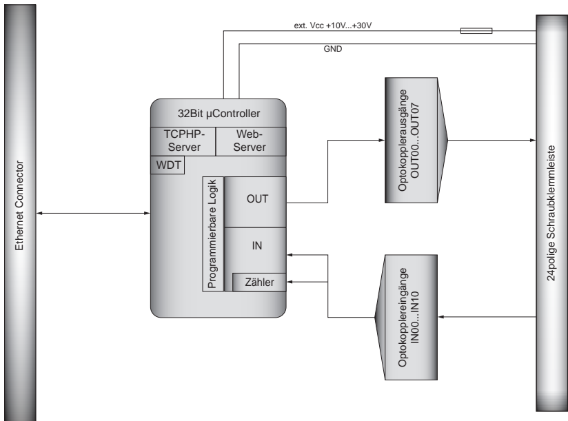
Grafik 3.2 Blockschaftbild EXDUL-519S
