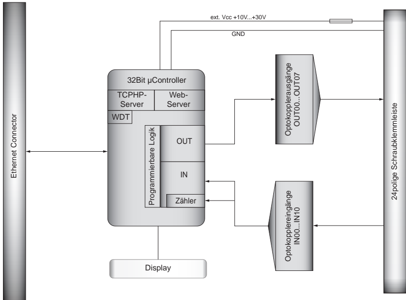
Grafik 3.1 Blockschahtbild EXDUL-519E
