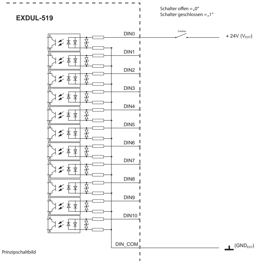
Grafik 17.1.1 Beschaltung der Optokopplereingänge
