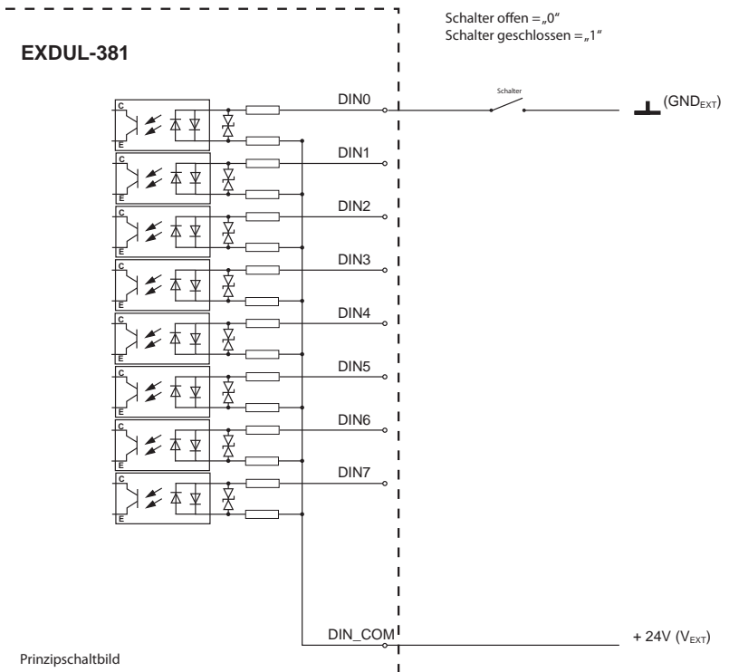
Graphik 13.1.2 Beschaltung der Optokopplereingänge revers
