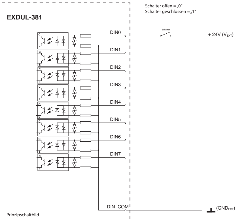
Grafik 13.1.1 Beschaltung der Optokopplereingänge
