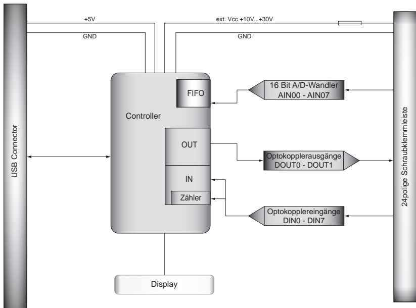
Grafik 3.1 Blockschahtbild EXDUL-381E
