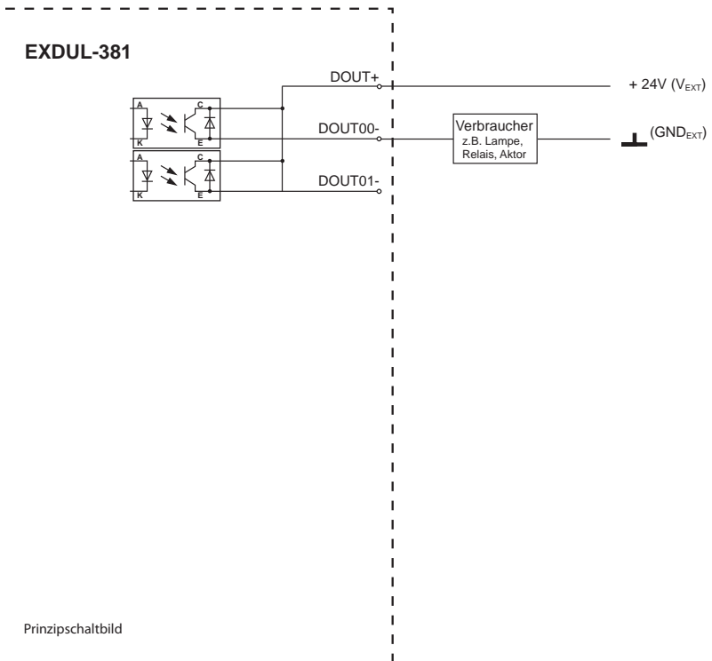
Grafik 13.2 Beschaltung der Optokoppler-Ausgänge
