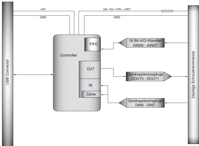
Grafik 3.2 Blockschahtbild EXDUL-381S
